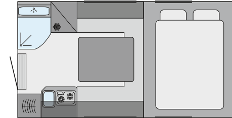
Inneneinrichtung TRAIL/BOX 240
